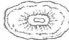
3. Fissurella crassa
