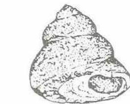
14. Tegula atra
