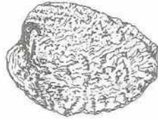
2. Concholepas concholepas
