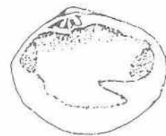
9. Protothaca thaca
